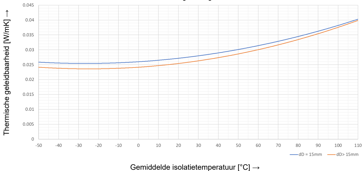
Warmtegeleidingscurve
