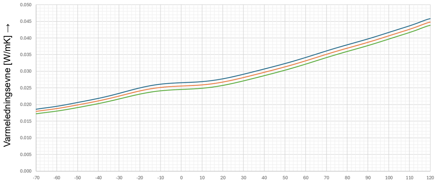
Termisk ledningsevnekurve: Tarepir M1-CR 33
