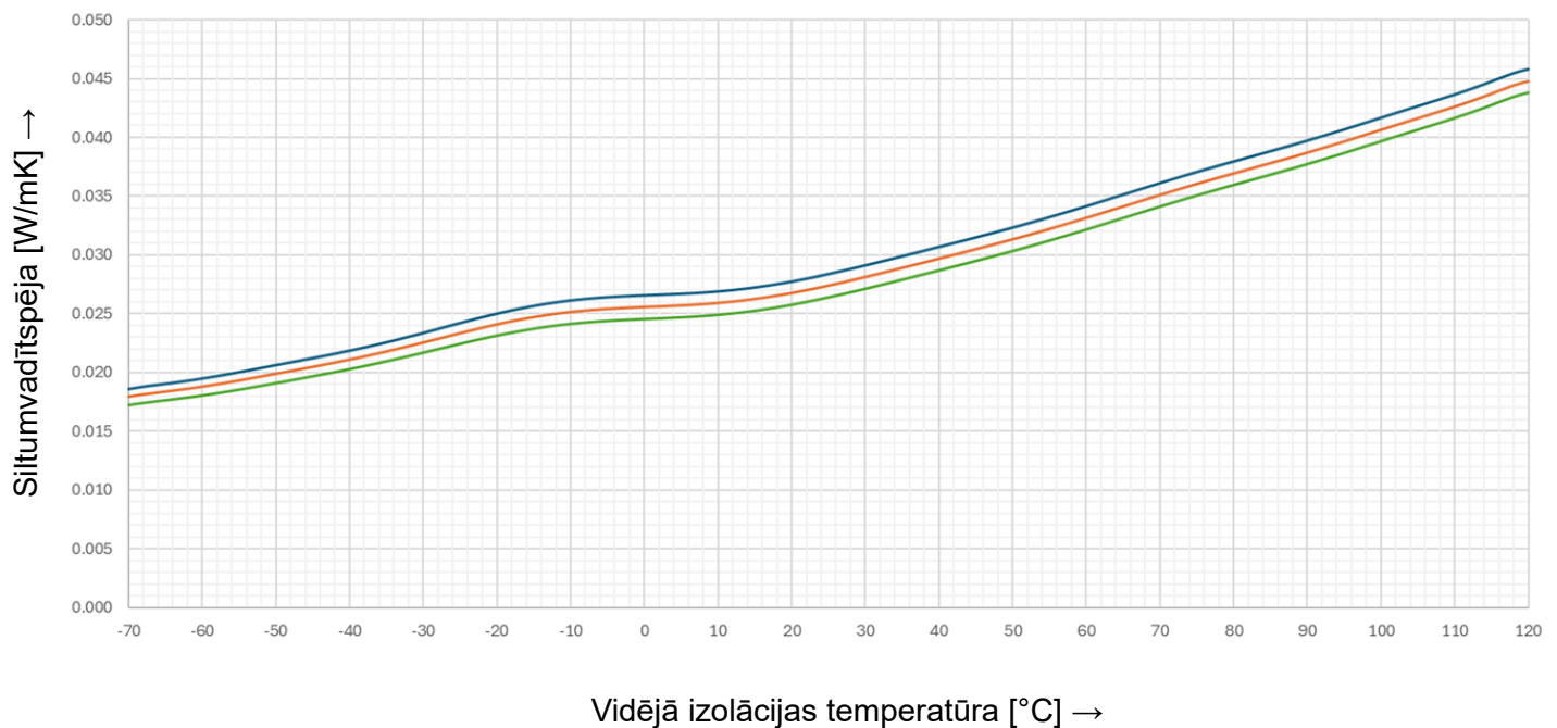
Siltumvadītspējas līkne: Tarecpir M1-CR 33
