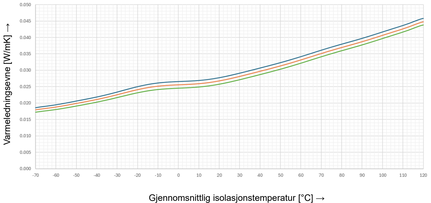
Kurve for varmeledningsevne: Tarepir M1-CR 33
