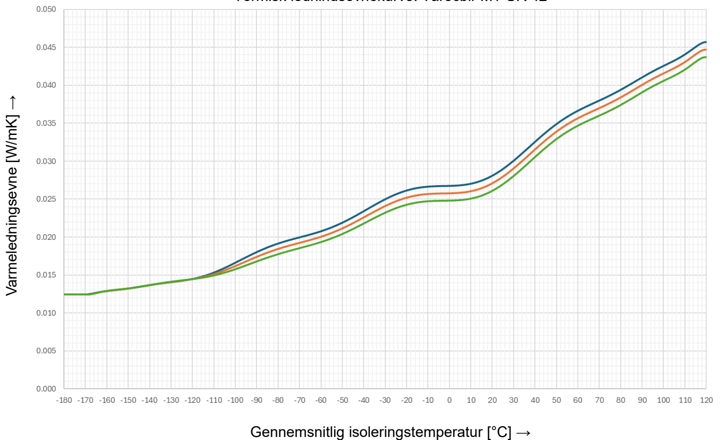
Termisk ledningsevnekurve: Tarecpir M1-CR 42
