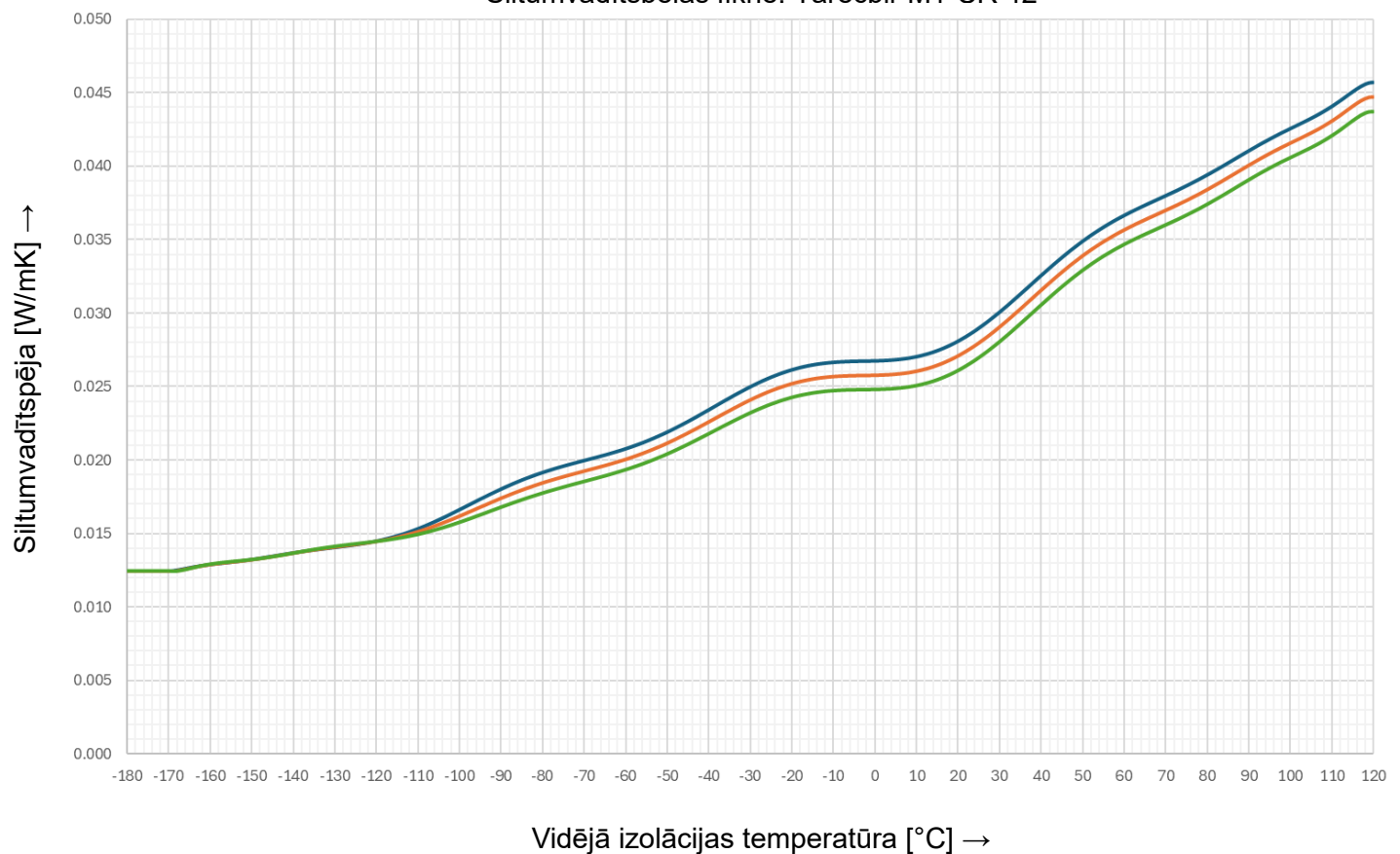
Siltumvadītspējas līkne: Tarecbr M1-CR 42
