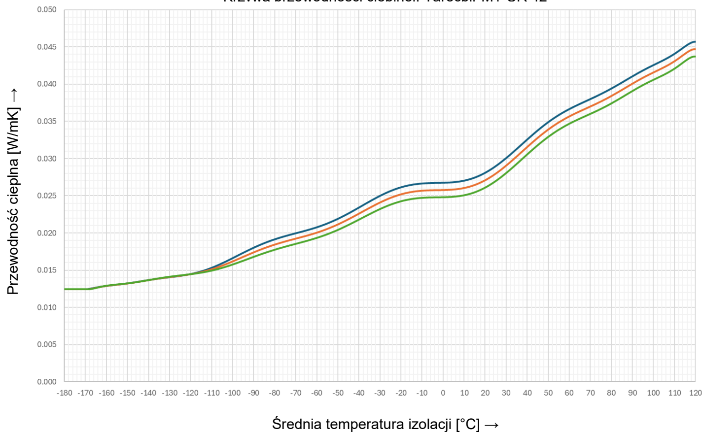
Krzywa przewodności cieplnej: Tarecdir M1-CR 42
