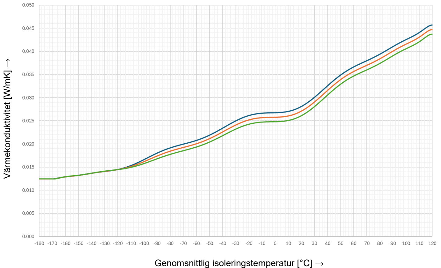
Kurva för värmekonduktivitet: Tarecpir M1-CR 42
