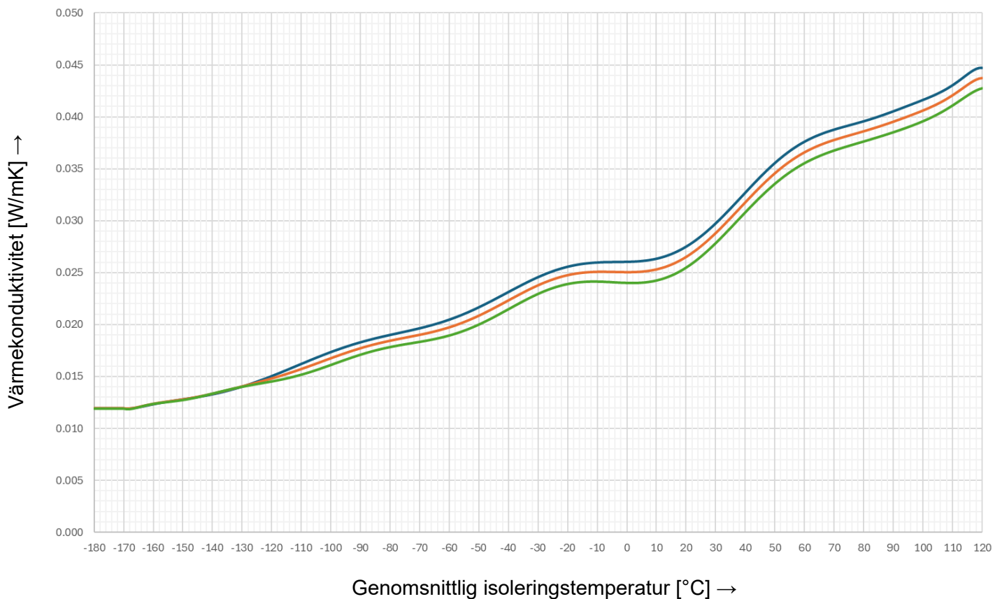
Kurva för värmekonduktivitet: Tarepir M1-CR 50
