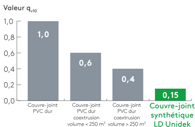
Graphique 2 - Comparaison du couvre-joint synthétique LD d'Unidek avec d'autres profils disponibles sur le marché
